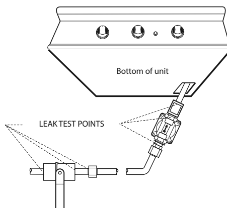
FIG. 16 Nat. Gas
