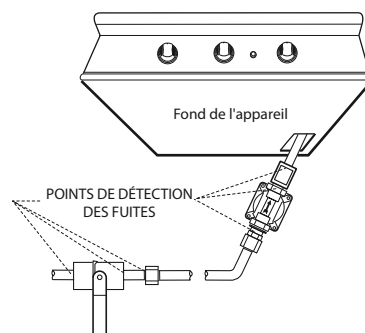
FIG. 16 Gaz naturel
