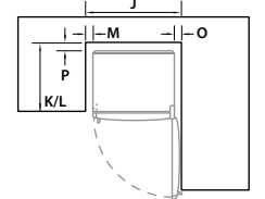
3. Flush with refrigerator door – 90° door rotation*
