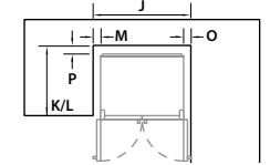
3. Flush with refrigerator door – 90° door rotation*
